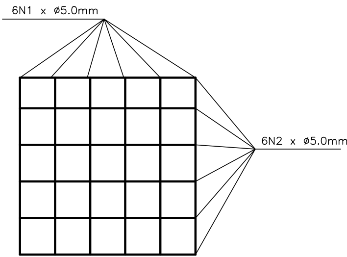
FERRAGEM DA TAMPA
