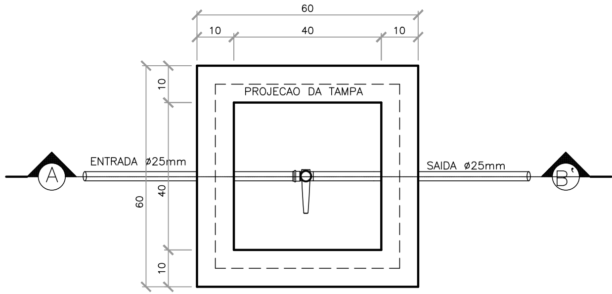
PLANTA BAIXA
