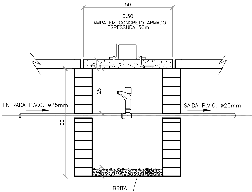
DETALHAMENTO CAIXAS DE PASSAGEM ESCALA: 1/10
