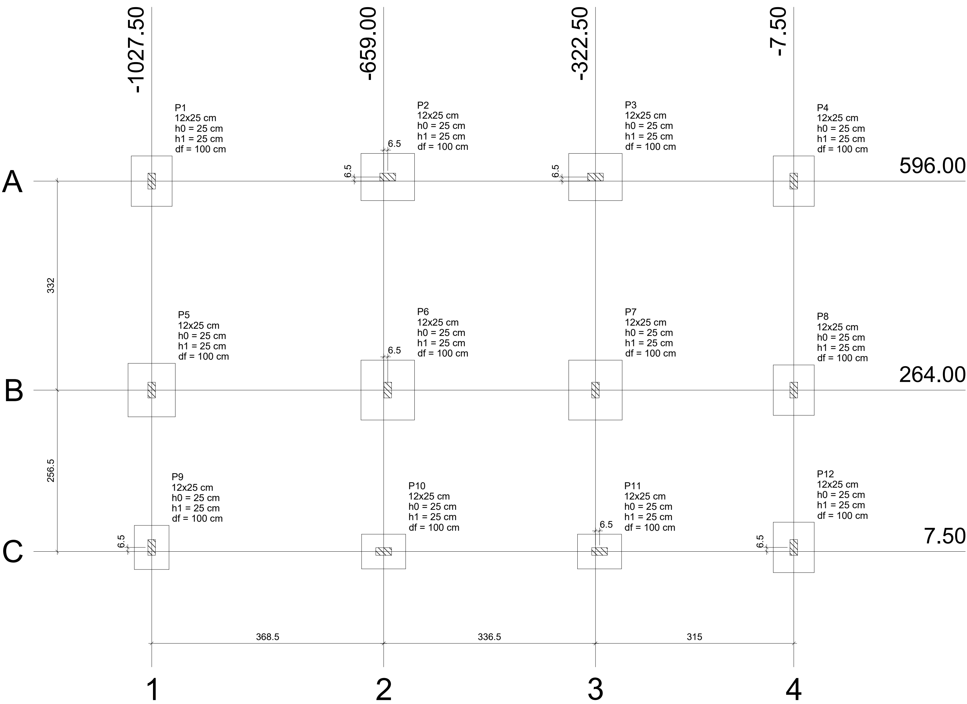
Planta de locação escala 1:75
